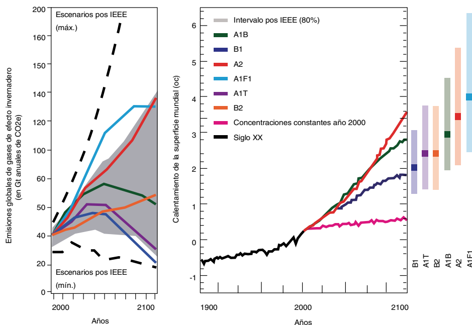
Gráfico I.8 ESCENARIOS DE EMISIONES DE GASES DE EFECTO INVERNADERO EN 2000 Y 2100 (EN AUSENCIA DE POLÍTICAS CLIMÁTICAS ADICIONALES) Y PROYECCIONES DE TEMPERATURAS DE LA SUPERFICIE
