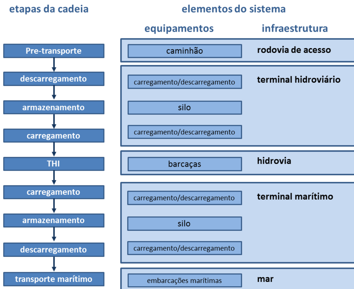
Figura 4.3 - Cadeia de Transporte Hidroviário Interior entre Origem (região produtora) e Destino.
